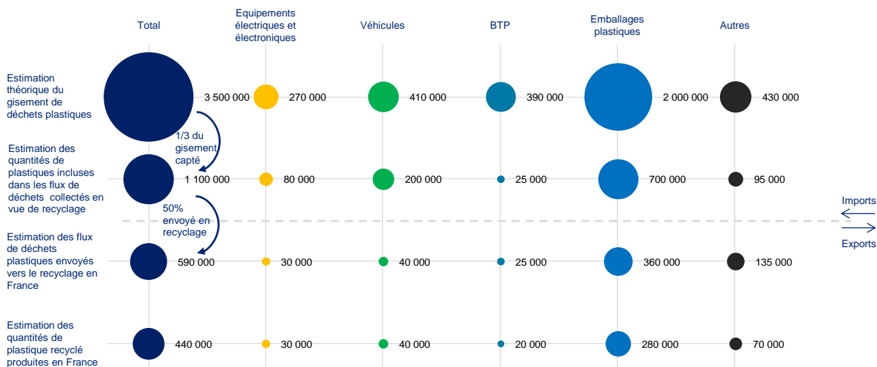
Figure 10 - Flux de déchets plastiques en France par origine (tonnes) - 2012
