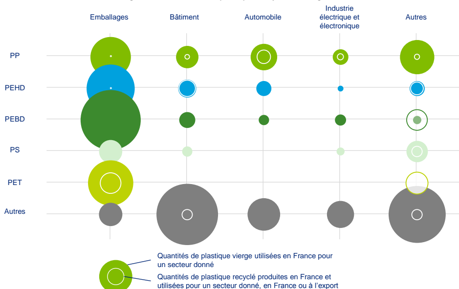
Figure 29 - Utilisations de plastiques recyclés et vierges - 2012
